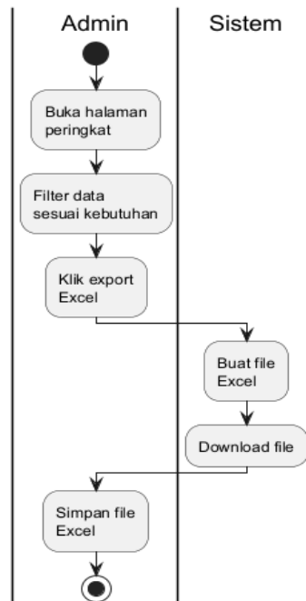
Gambar IV.12 Activity Diagram Ekspor Peringkat
